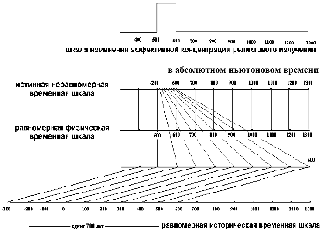
Рис. 1. Пример различных шкал времени и сдвига исторических и физических датировок в зависимости от изменения эффективной концентрации реликтового излучения
